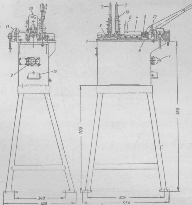
圖 1 АСП-3型對焊機外形圖
