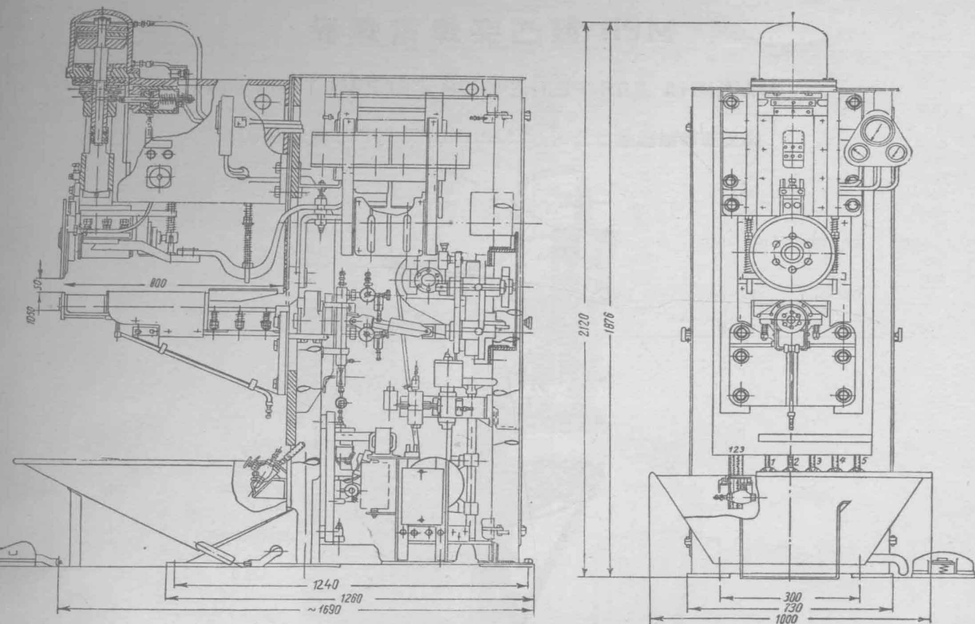
圖 2 MSH-150-1 型電焊機外形尺寸圖
