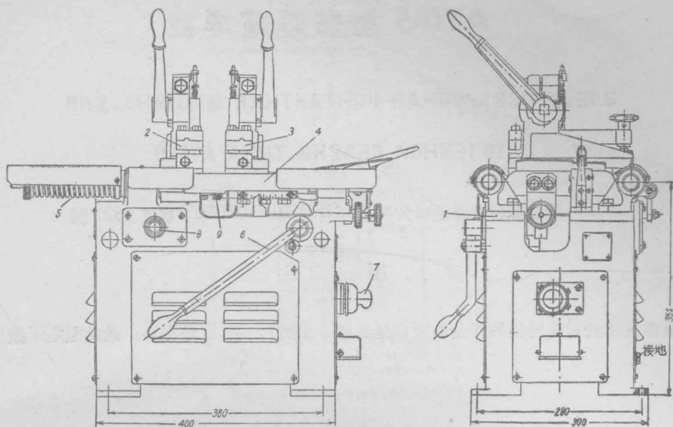
圖2 АСИФ-5型對焊機外形圖
