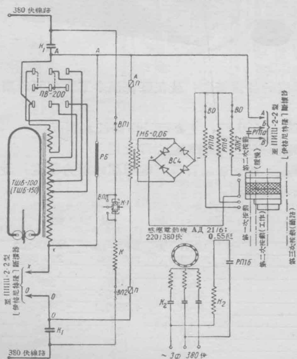
圖 3 電焊機結線圖
