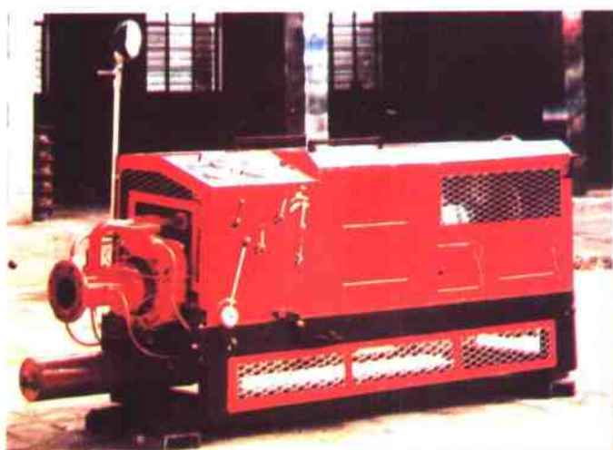
BDG40/100固定式消防泵组
