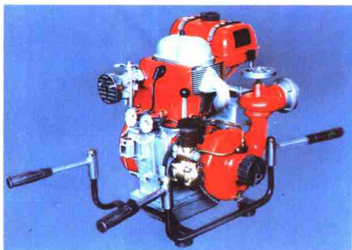
BJ10A型手抬机动消防泵
