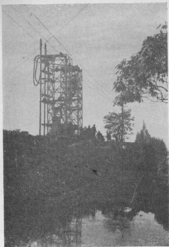
▷闽江防洪堤洪山段土堤防渗样施工
