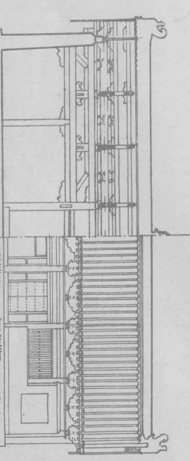
佛光寺文殊殿纵断面
