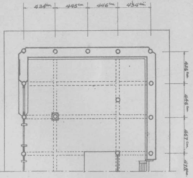
山西五台山佛光寺文殊殿平面
