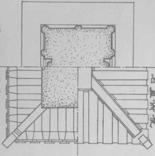
石屋平面
