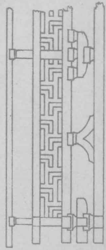
金堂欄杆立面圖
