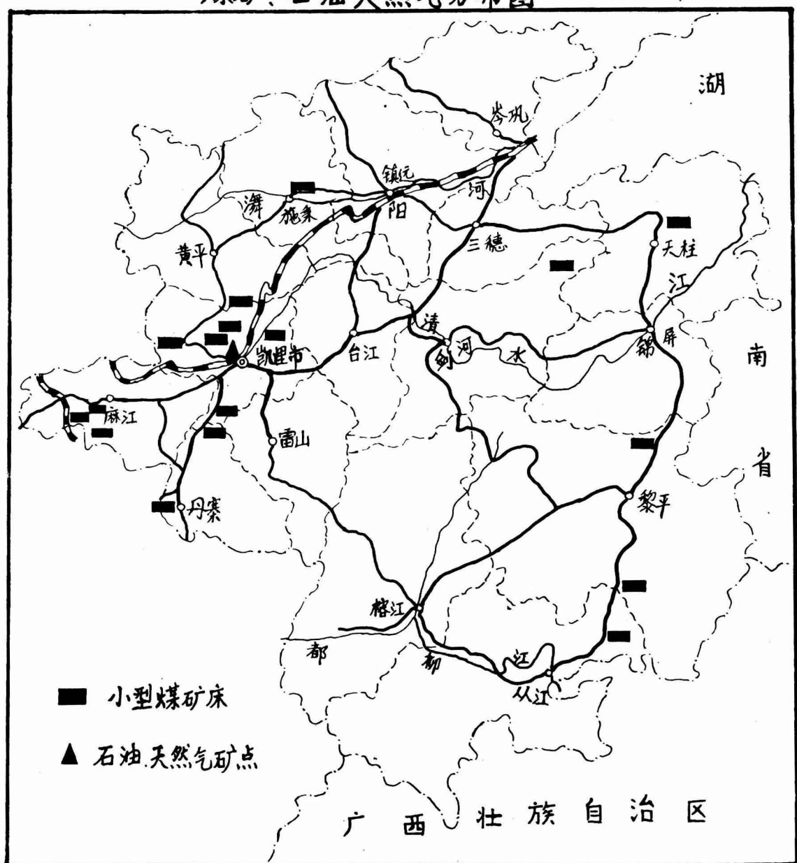
煤矿、石油天然气分布图
