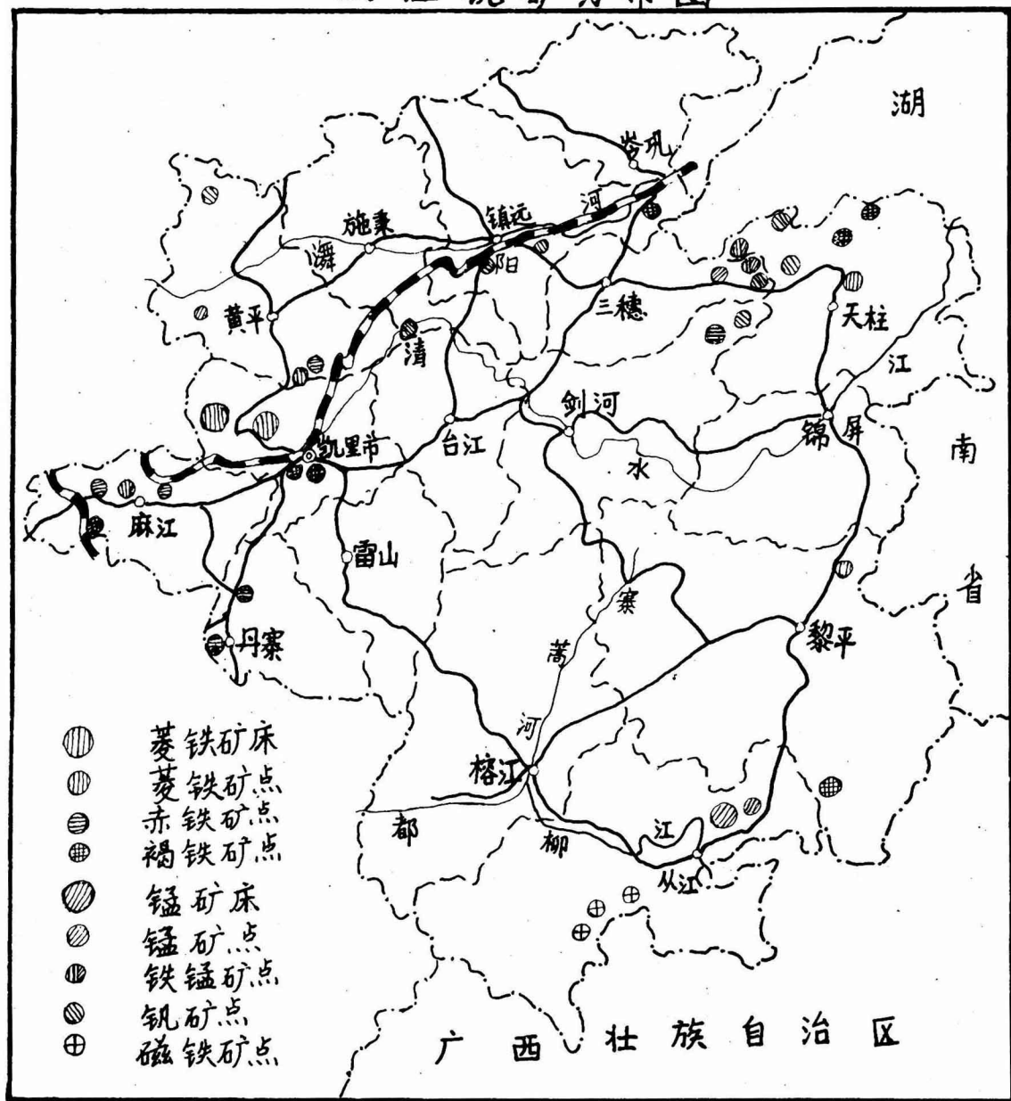
铁 锰 钒 矿 分 布 图
