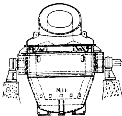
图3 风口部分和旋转轴承的高度图
