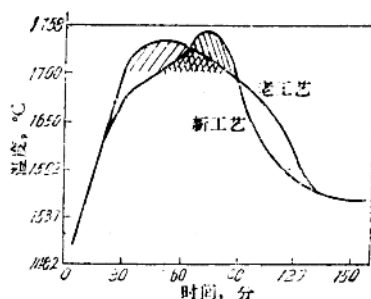
图 9 正确的吹炼工艺可大大缩短耐火材料在 3100°F 的暴露时间
