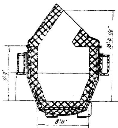
图2 炉子横断面图
