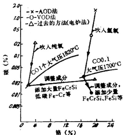
各种操作法的成分变化 (304L)
