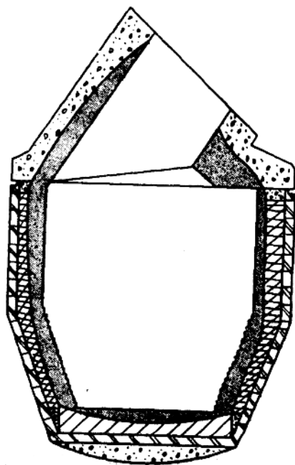
图8 现在炉子均匀侵蚀的典型图
