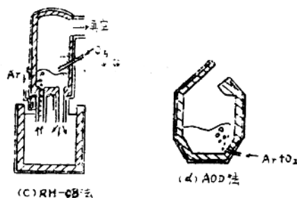
图3 各种二次精炼炉的原理图
