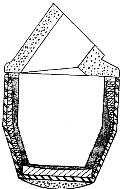
图6 说明风口和风口炉壁问题的初期炉子侵蚀图 所有侵蚀图形均通过风口中心的断面
