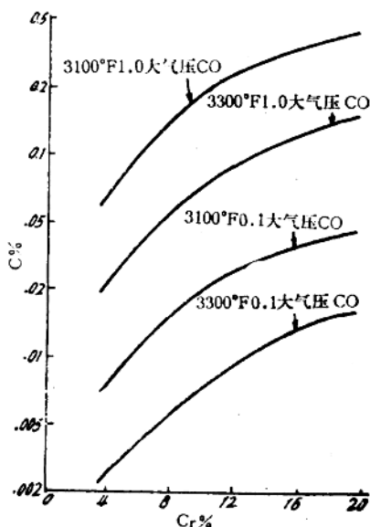
图1 碳-铬平衡关系是温度和压力的函数
