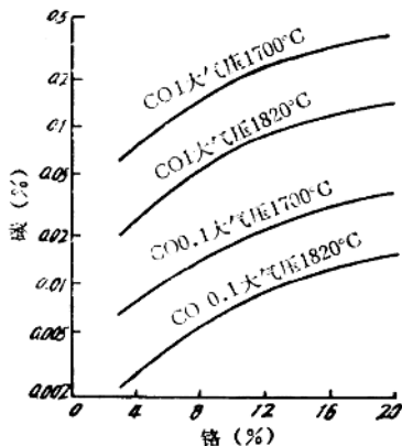
图 1 碳-铬平衡关系
