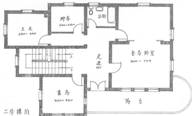
三層樓面
