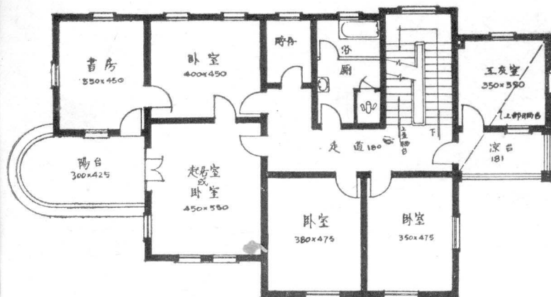
樓層平面
