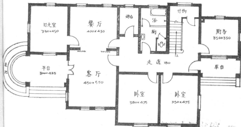
底層平面
