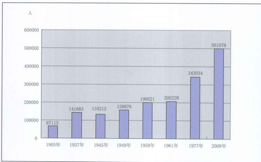
图1 清镇市几个时期总人口比较图
