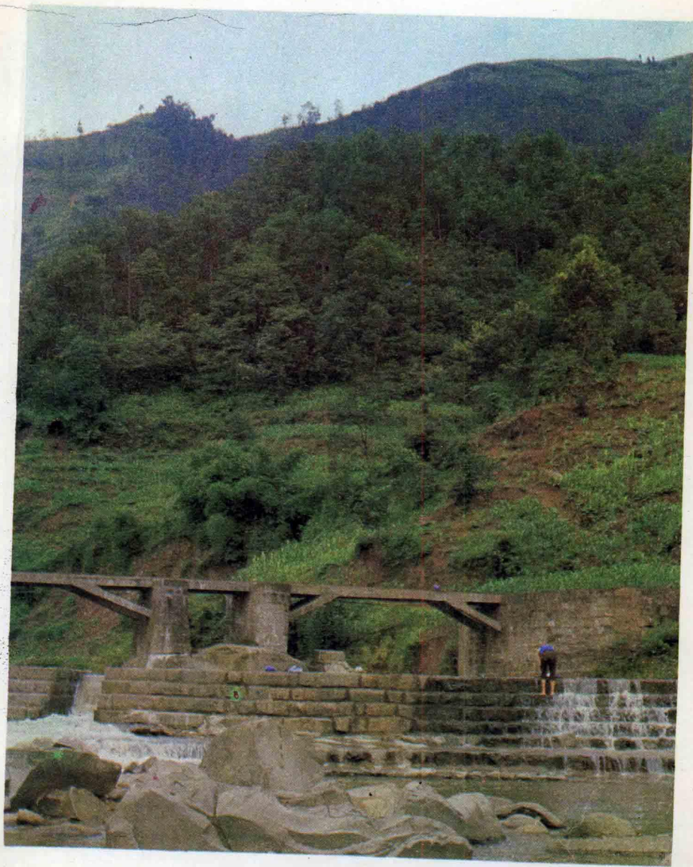
盐津建兰生境图
