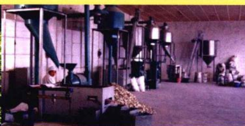
魔芋精粉加工生产线一角
