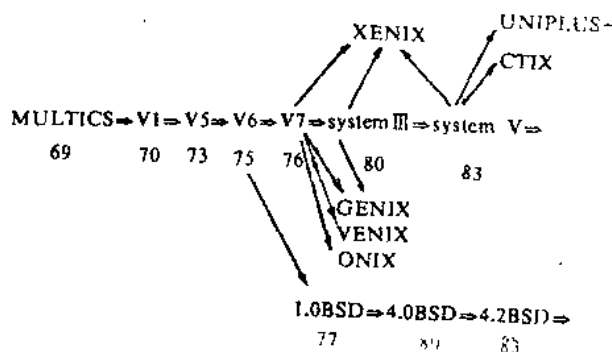
图 2.1 UNIX 系统的演变
