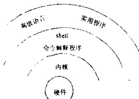
图 2.2 XENIX 系统概貌和结构
