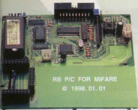
多力MIFARE标准万用开发板RB-P/C
