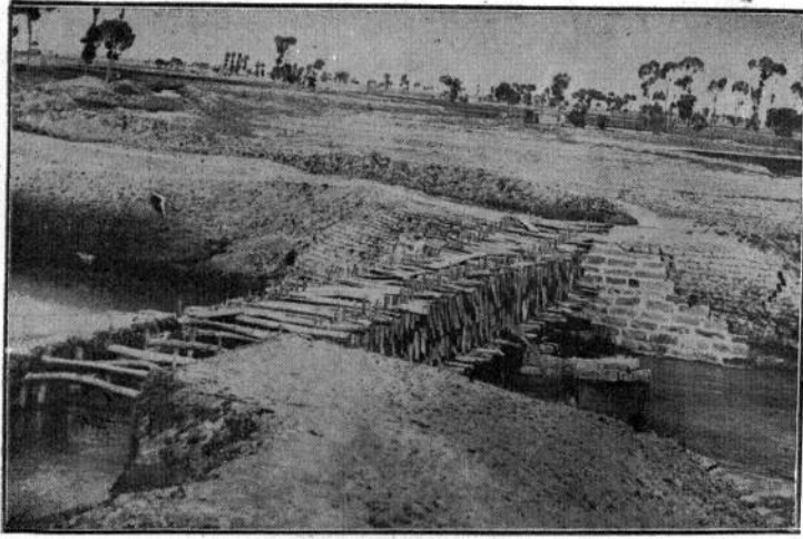
● 惠農渠方家巷之跳水壩
