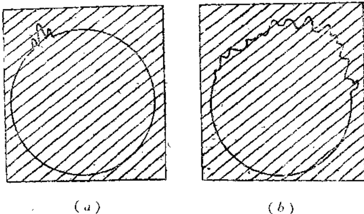
图9.1 受铝箔条干扰前后圆扫描显示器画面的图形
