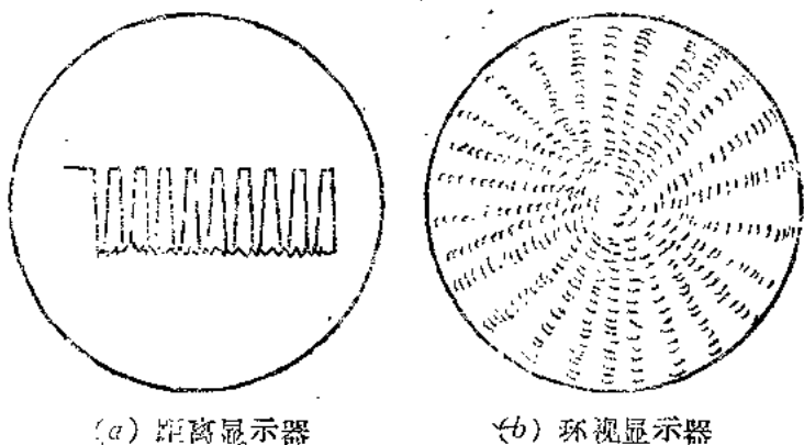
图 9.4 高频正弦调幅干扰在显示器画面上的图形
