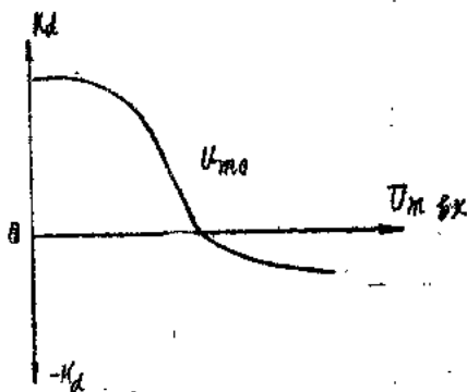
图 9.9 增量放大量与输入电压振幅的关系图
