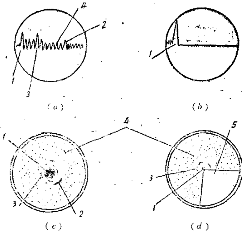
图9.2 等幅波干扰使接收机过载时,雷达显示器的画面图 (a)、(b)为干扰前后的距离显示器, (c)、(d)为干扰前后的环视显示器。
