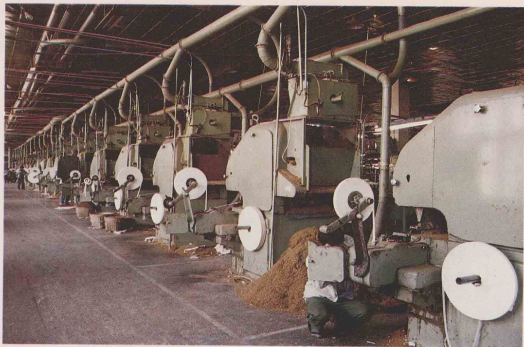
昭通卷烟厂七十年代的制丝设备
