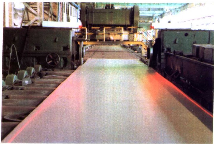
圆盘剪激光标线装置
