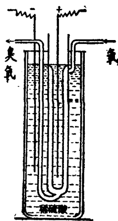
圖五 製造臭氧 的裝置
