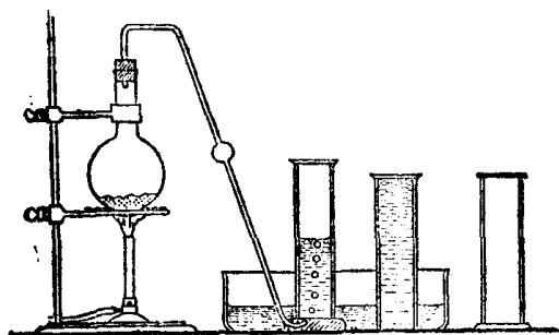
圖三 氧的捕集
