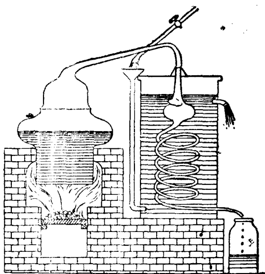
圖八 大規模的水的蒸餾裝置
