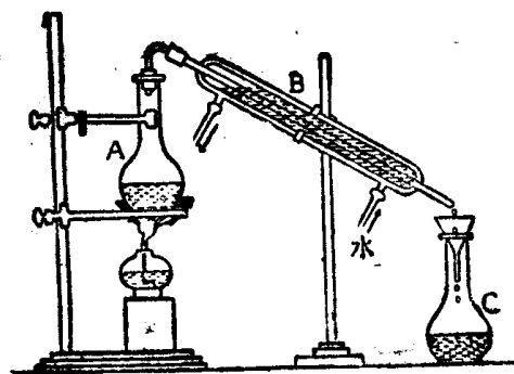
圖七 水的蒸餾裝置 A瓶中的水加熱沸騰，水蒸氣通過冷卻器 B之後，凝縮為純水而滴入C瓶
