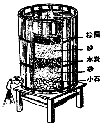
圖六 家庭濾水器橫斷面 表示內部材料的充填法
