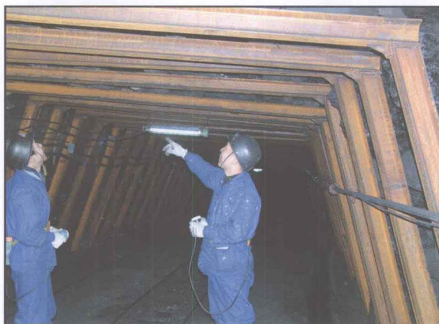
井下使用的钢制箱架
