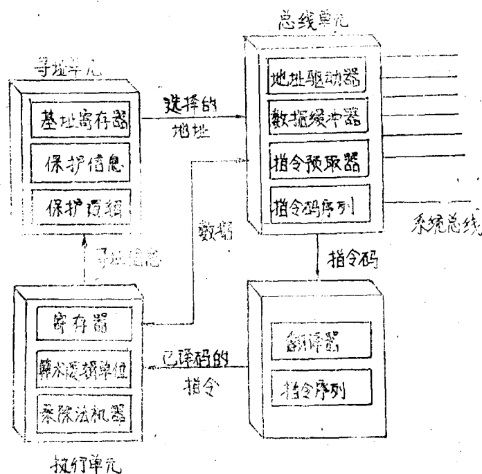
图1-2 80286框图
