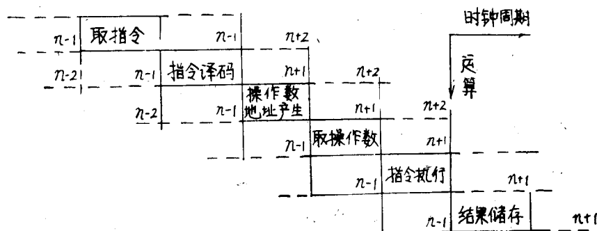
图1-1 80286指令总线
