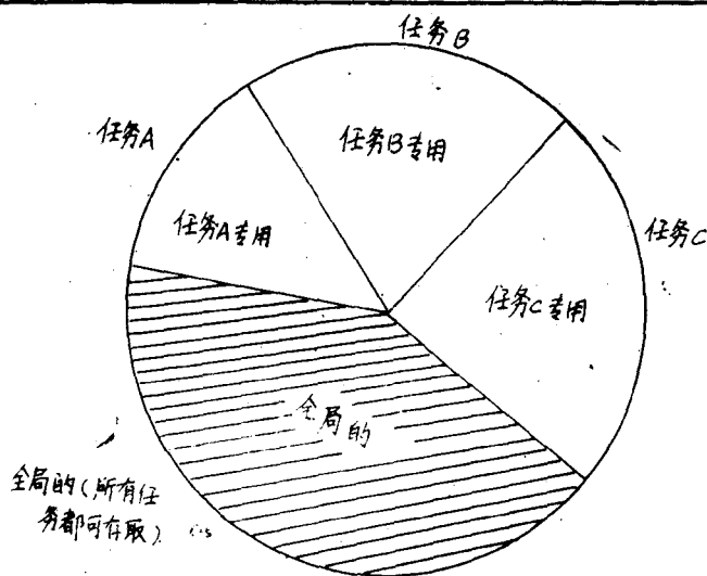
图2-2 存在80286系统内的“多任务”
