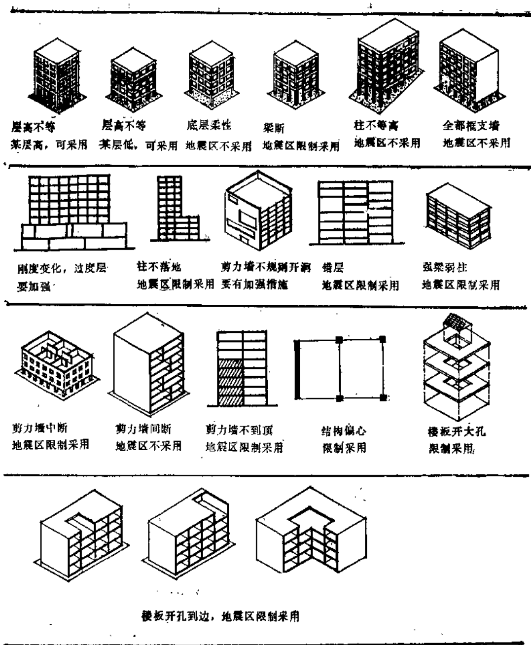
图1-8 不规则结构布置示例
