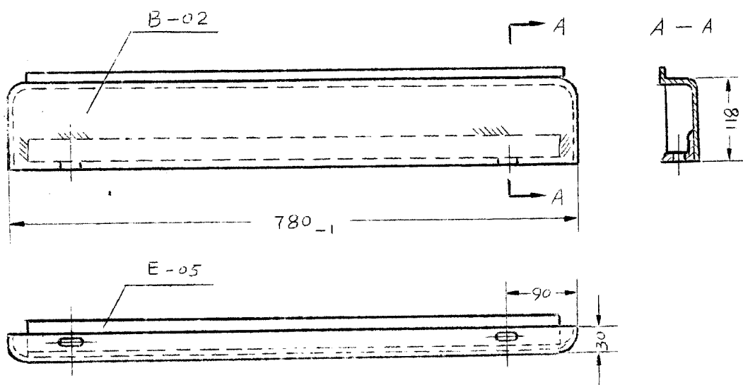
底 框 架
