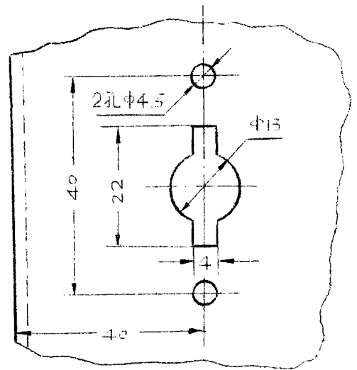
门锁开孔图
