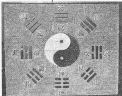
图4 先天八卦图
