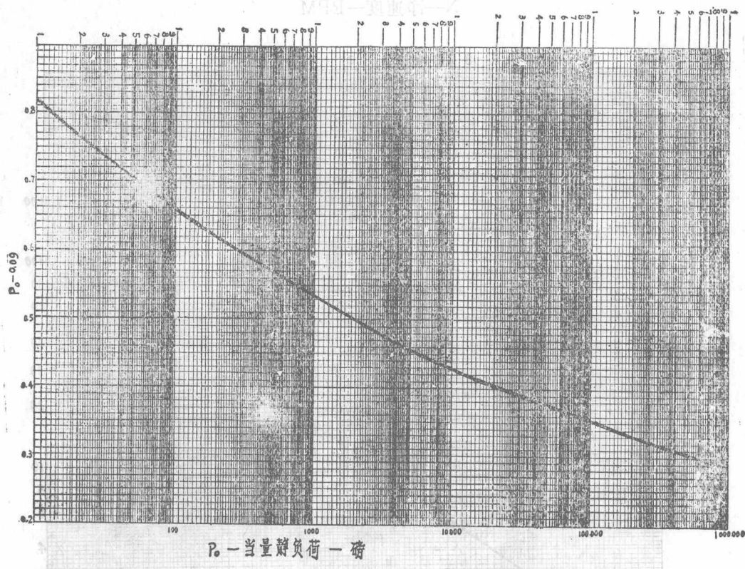
图 8 与 P_0 对应的 P_{0-0.09} 值
