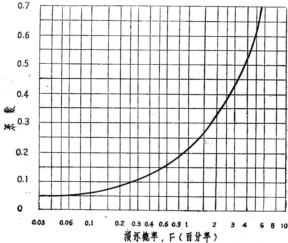
图4 寿命的可靠性调整系数
