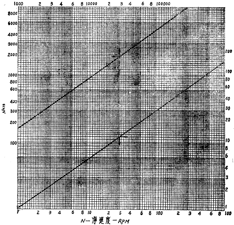
图 7 与N对应的 N^{0.73} 值
