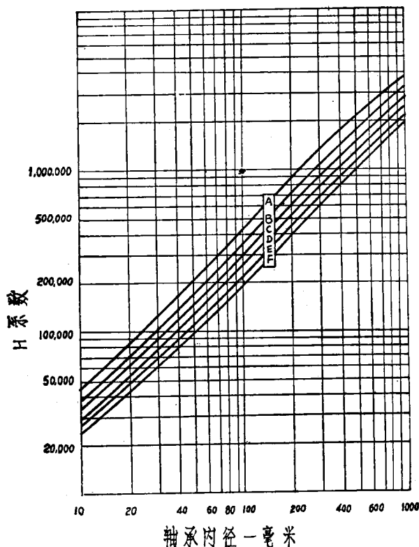
图 5 与SKF各系列轴承内径对应的H系数
