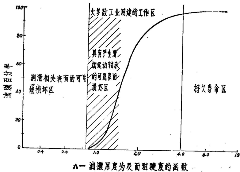
图 9 与 \Delta 对应的油膜百分率
