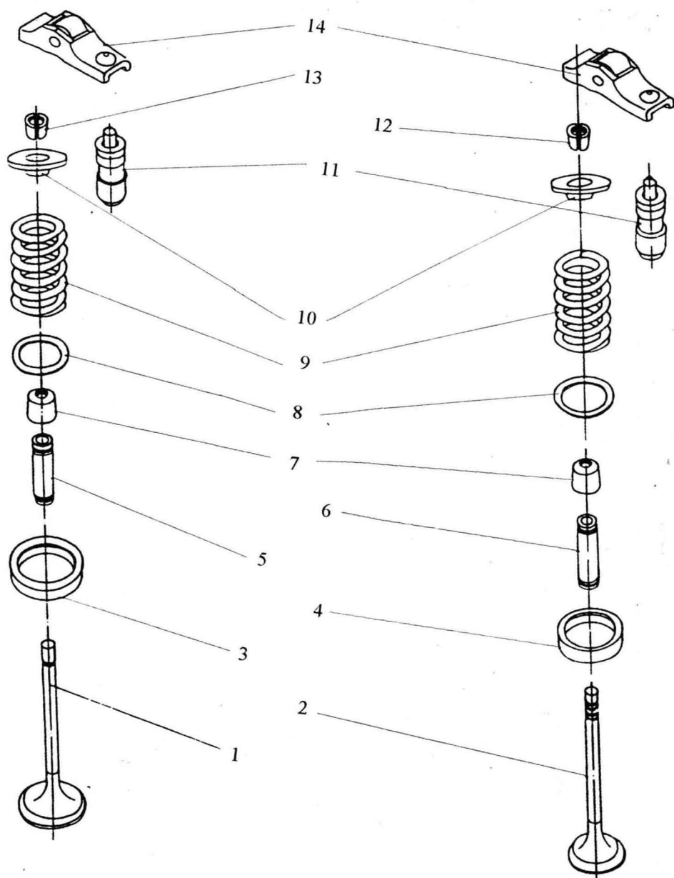
图 4 气门机构
