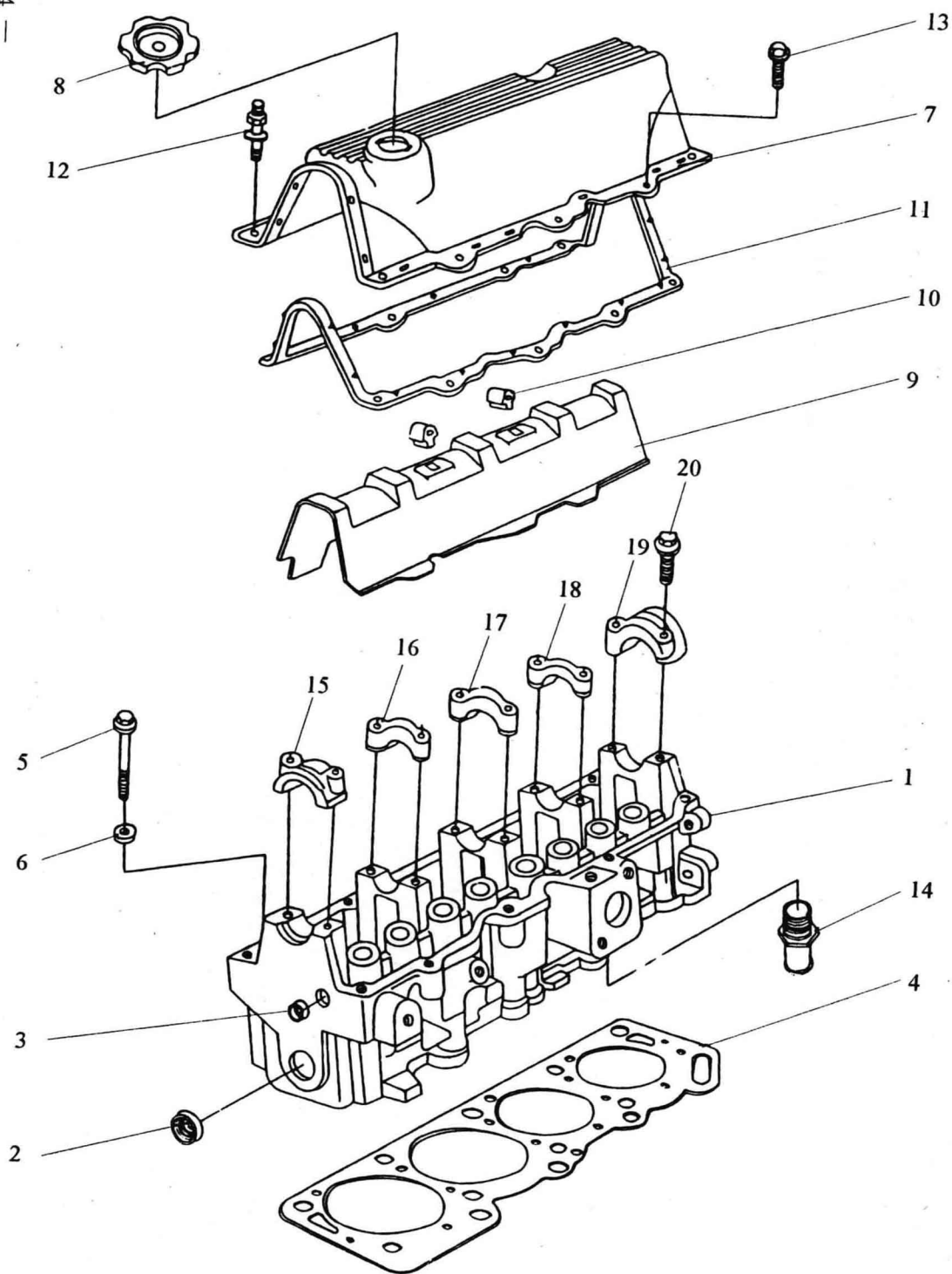
图 2 气缸盖
