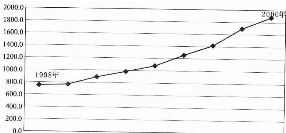
规模以上工业增加值 (亿元)
