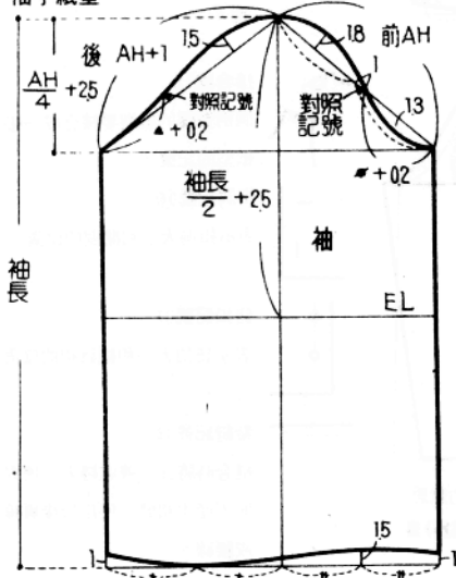
袖子紙型
