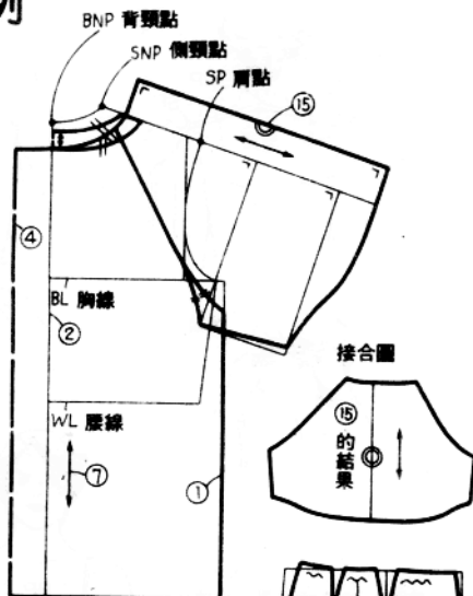
褶襞的方法
