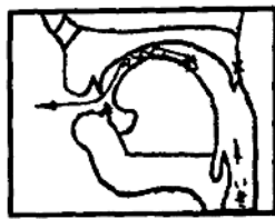
[ʃ] 图 11
