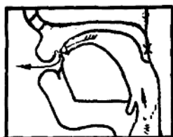
[s] 图 10
