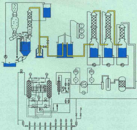
RYQ-40/80型溶解乙炔设备工艺流程图
