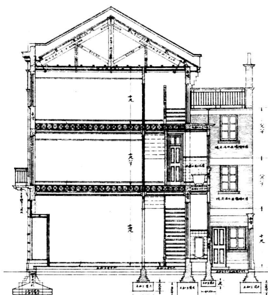
剖面
