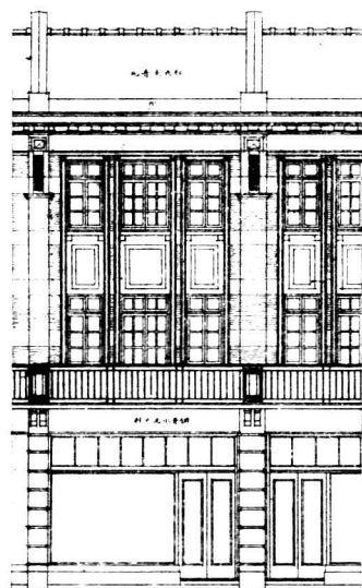
正面
