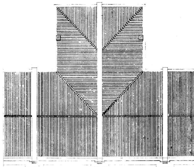
屋頂平面圖
