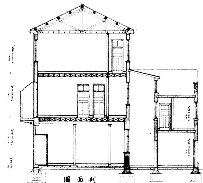
圖面側
