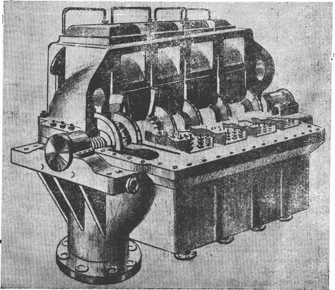
图 0—3 等温型离心式压缩机
