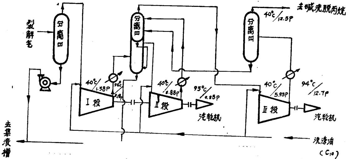
图 0—7 裂解气压缩流程示意图
