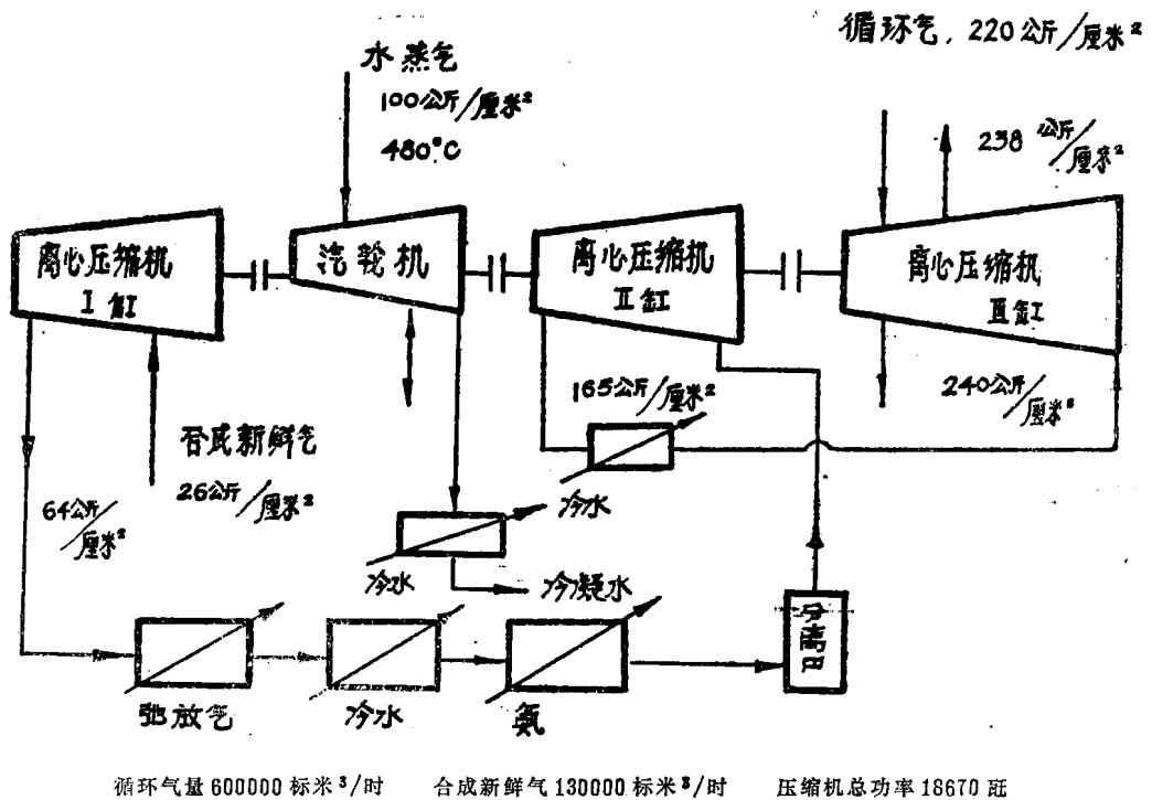
图 0—5 合成氨厂氮氢合成气压缩机系统示意图
