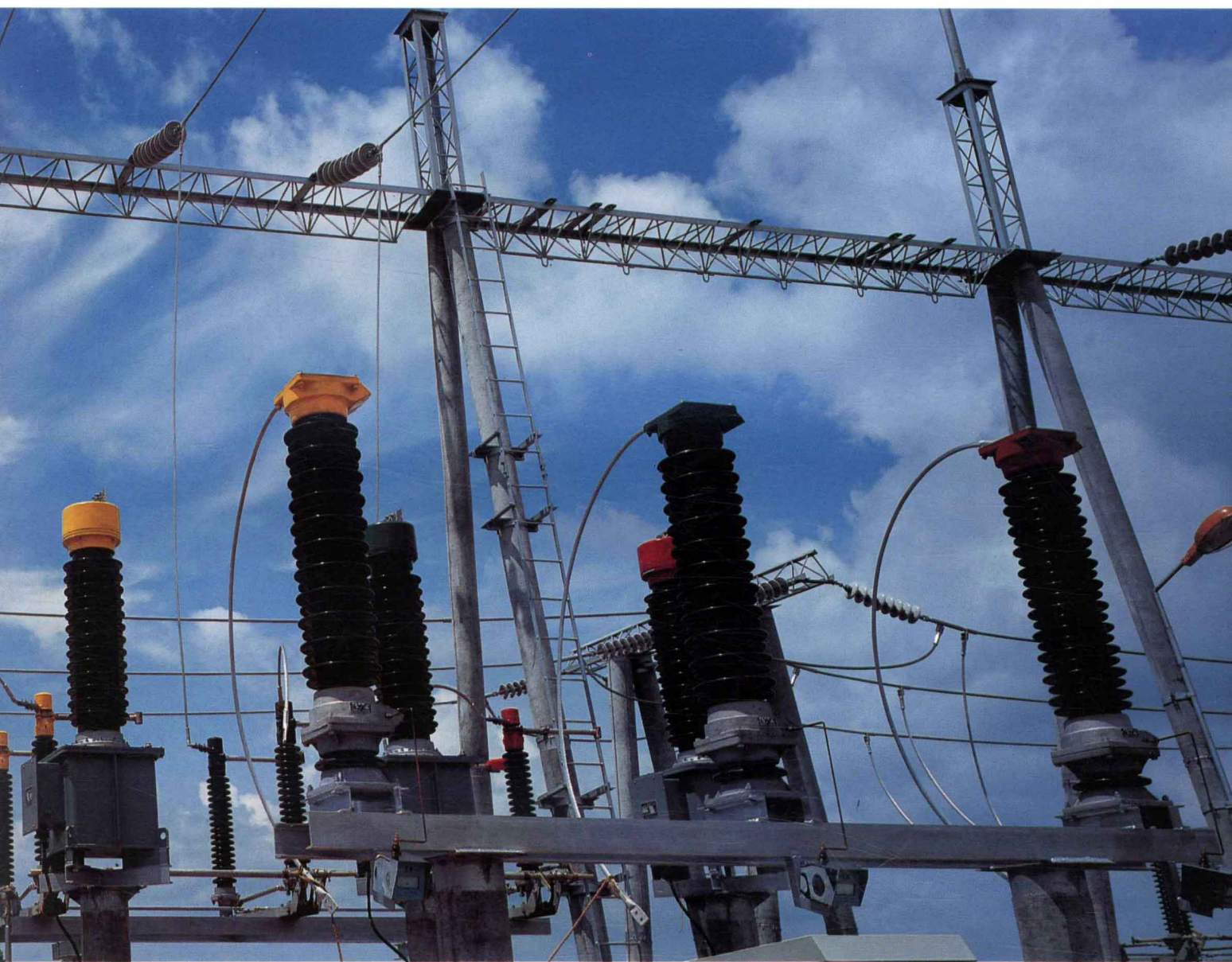
建设中的220千伏变电站
