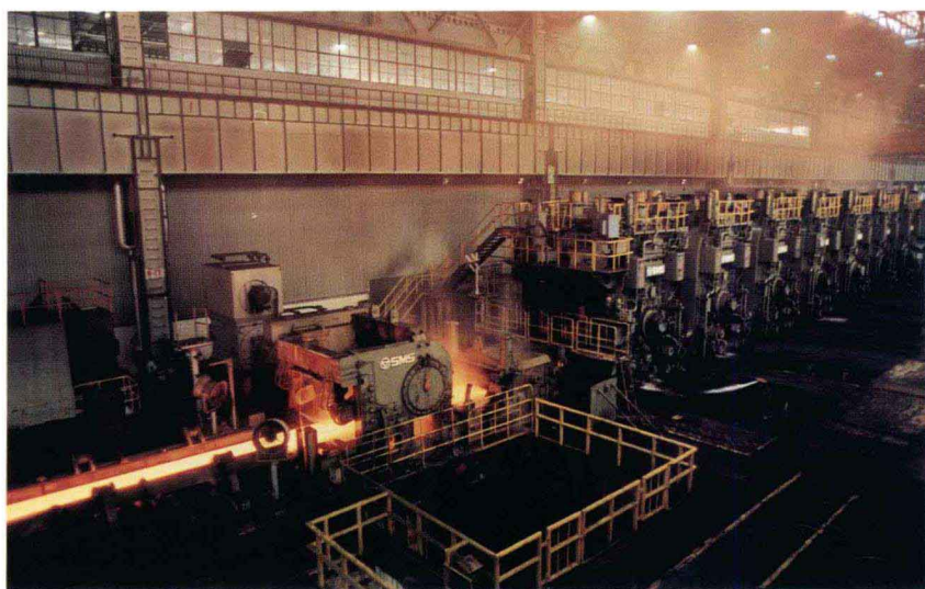
图为年产四百万吨钢卷的宝钢热轧厂（精轧机组）。热轧厂的全部生产过程由四级计算机控制。
