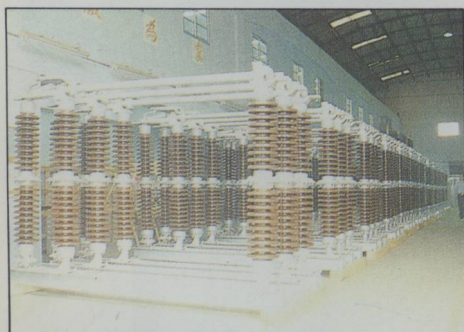
161KV 空斷開關 Air Breaker Switch
