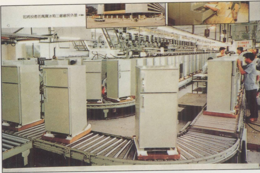
电冰箱及其装配线
