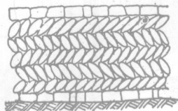
图6 竖砌石塘图
