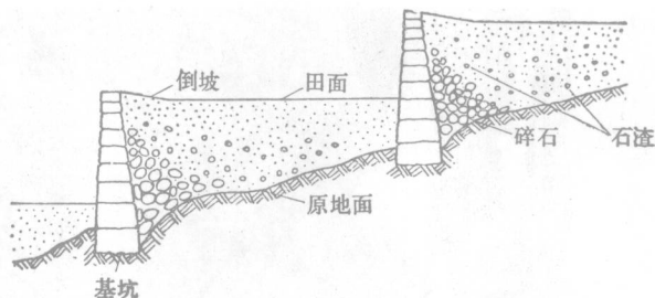
图3 单面石塘结构图
