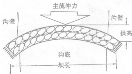
图8 拱形坝受力示意图
