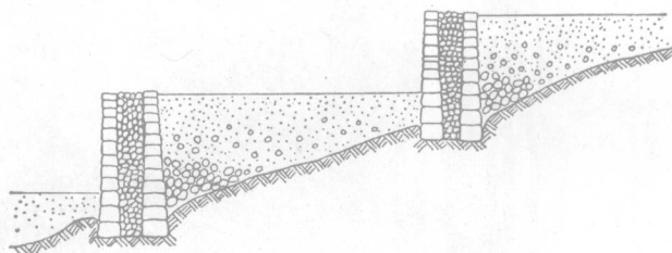
图4 双面石塘结构图
