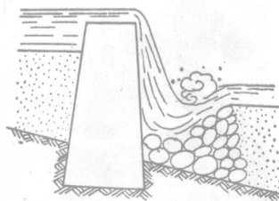
图9 跌水坑消力图
