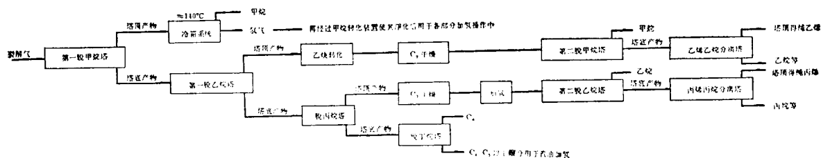
图 1—3 烯烃分离过程简图
