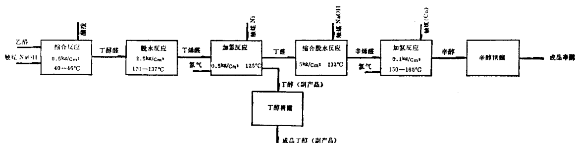
图 1—6 丁辛醇生产过程简图
