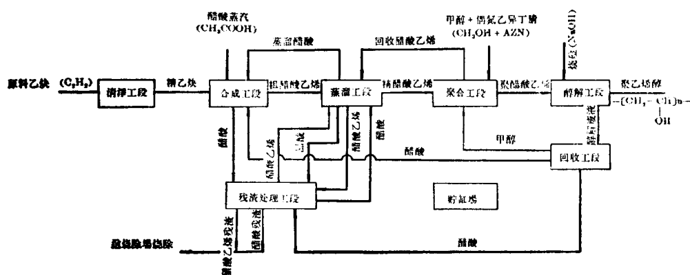
图 1—1 聚乙烯醇生产过程简图
