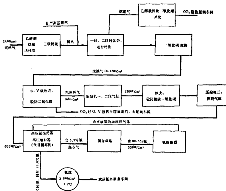
图 1—5 以天然气为原料生产合成氨的过程简图
