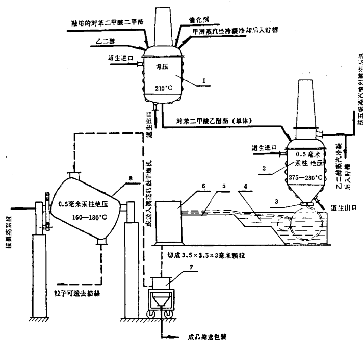
图 1—7 涤纶生产装置（聚合部分）主要生产过程简图
