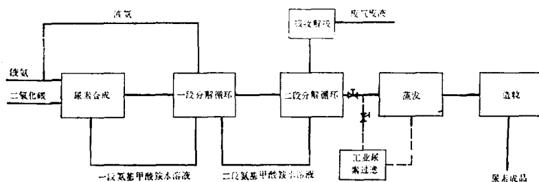
图 1—2 尿素生产过程简图
