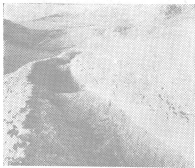
徽縣宏化鄉羣眾所作 的保土排洪溝
