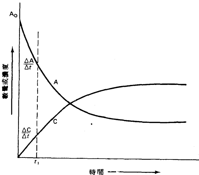
■ 2-1 在不同時間間段一反應中之一物質的濃度 (或數量) 圖。該反應如方程 5 所示，標記 A 的曲線代表方程 5 中品種 A 的濃度。標記 C 者代表此過程 C 的濃度。
