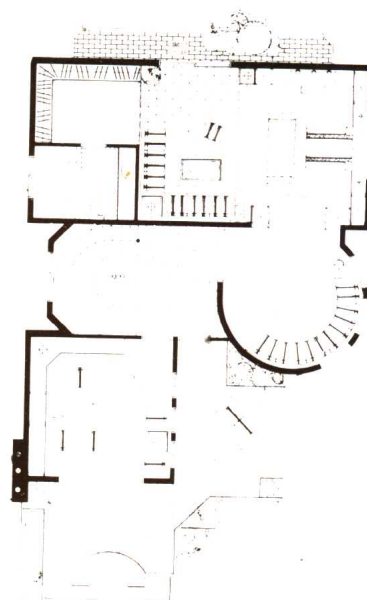
三樓平面圖
