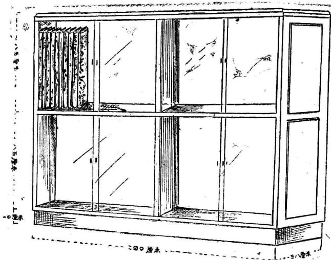
圖102. 有門貨櫥
