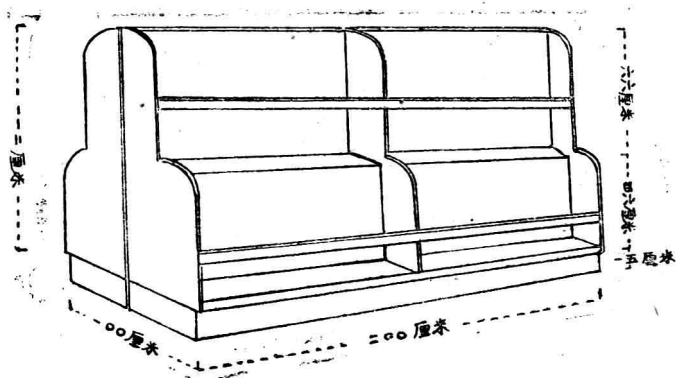
图104. 棉布貨架
