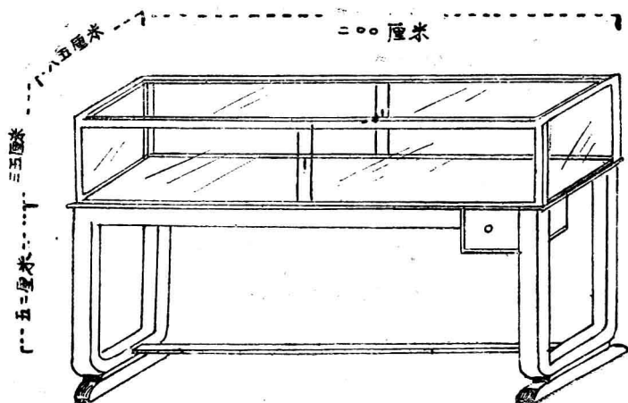
图100. 玻璃工作台
