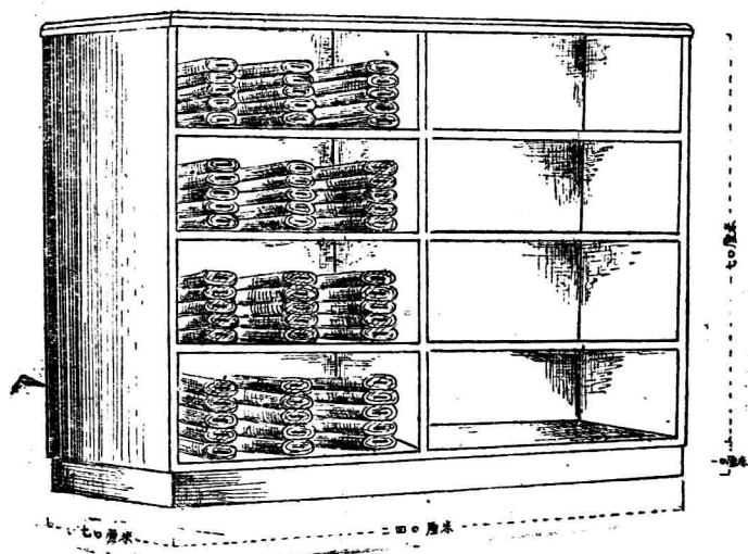
图101. 无門貨櫥
