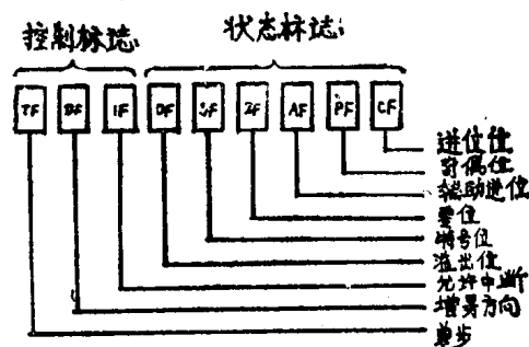
图 1-1-3 标志寄存器
