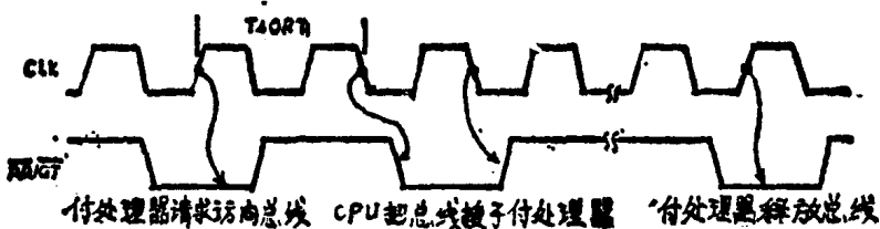
图 1-3-2 请求/授予的定时波形
