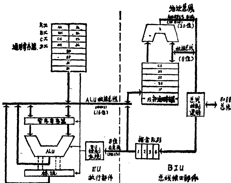
图 1-1-2 8088的基本结构方块图
