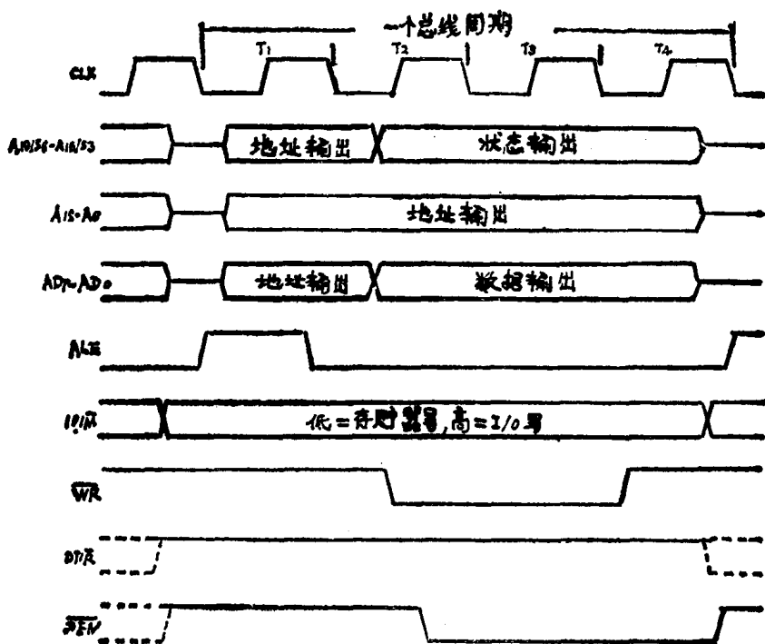
图 1-2-3 8088的写总线周期
