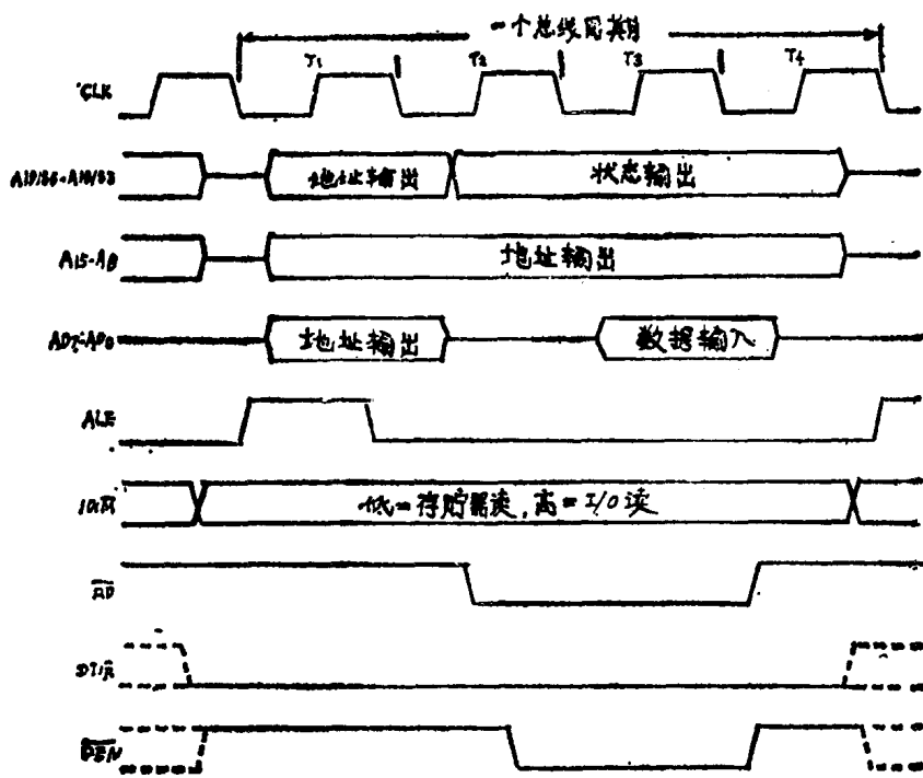
图 1-2-2 8088的读总线周期
