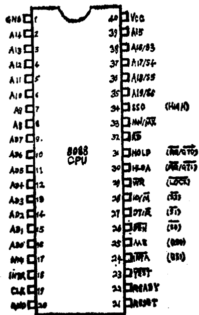
图 1-1-1 8088CPU的管腿说明 图中加括号的是最大方式管腿功能
