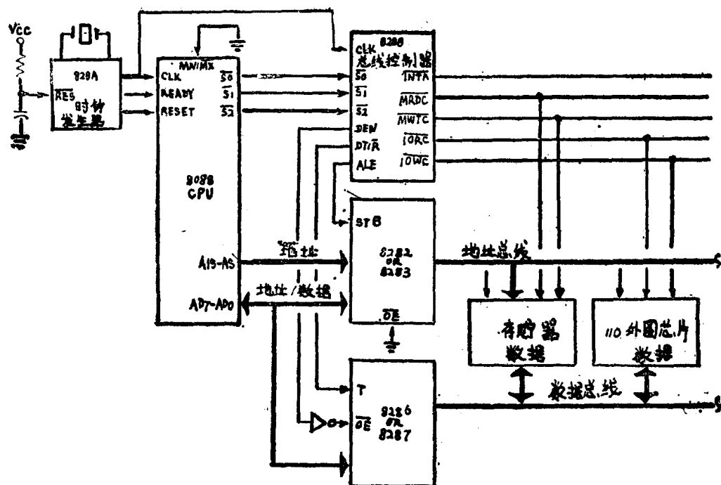
图 1-3-1 基本的最大方式系统
