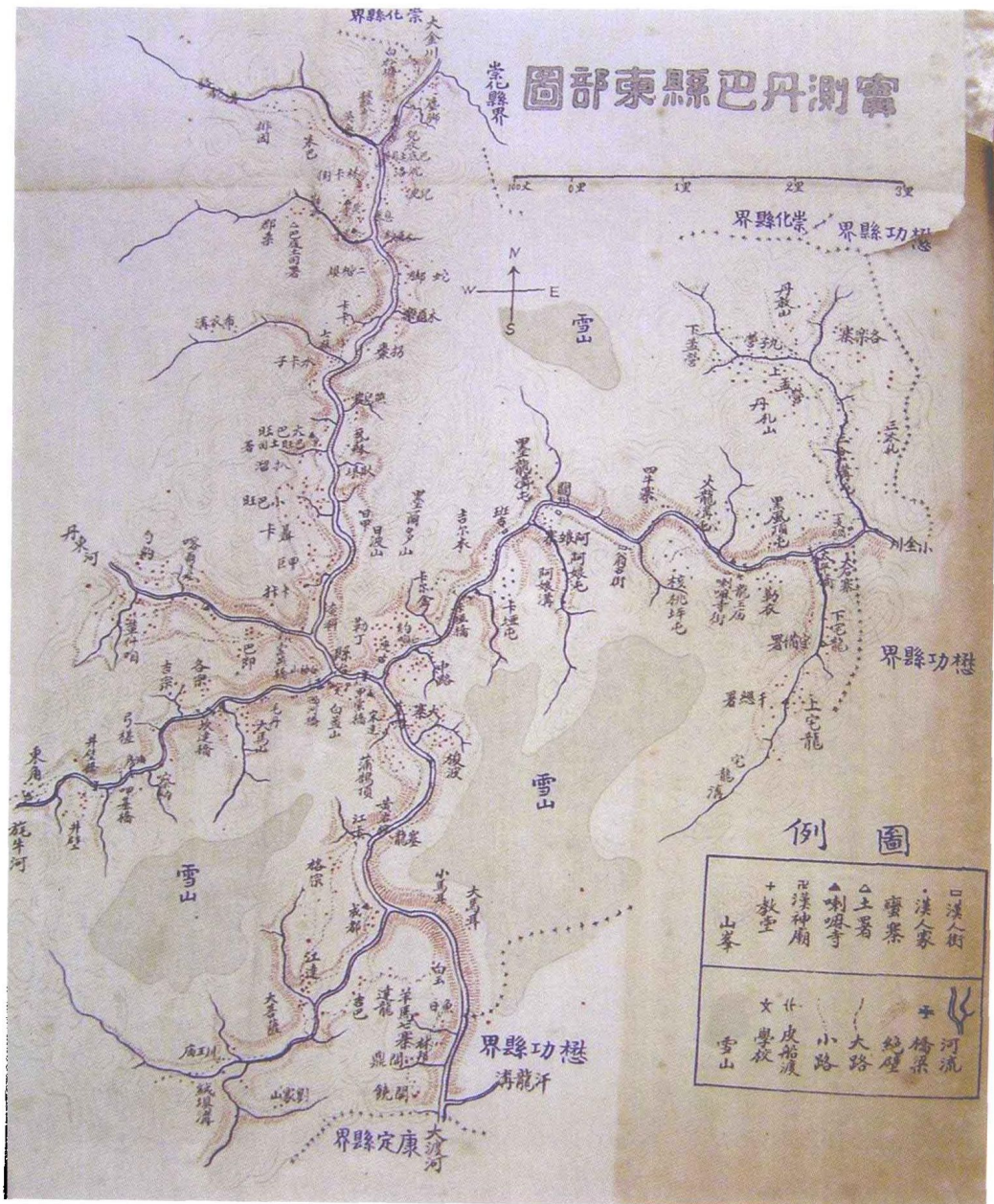
图4 实测丹巴县东部图
