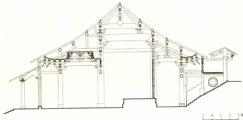
保国寺大殿剖面图
