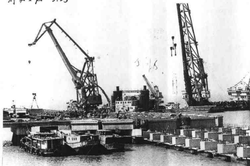
上海今年30项重大工程之一的外高桥港区3期码头建设，在完成了前期准备后，近日投入施工，工程将于今年10月竣工。图为三航202处职工正在水上作业。·本报记者 吴文腾 摄·
