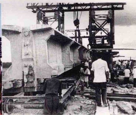
△桥梁预应力 T 梁安装
