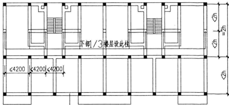
构造柱布置示意图 2
