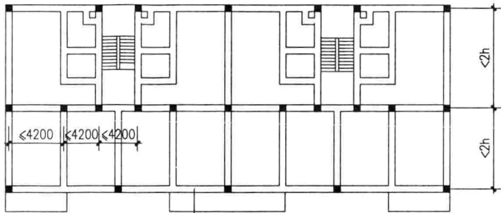
构造柱布置示意图1 层高 h
