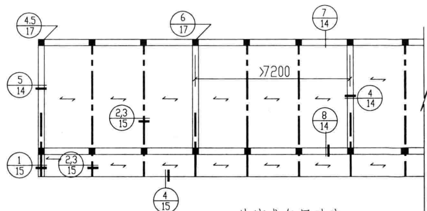
外廊式多层砖房
