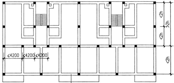
构造柱布置示意图3 层高 h
