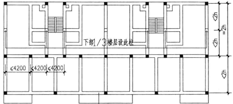
构造柱布置示意图2 层高 h
