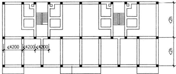
构造柱布置示意图 1
