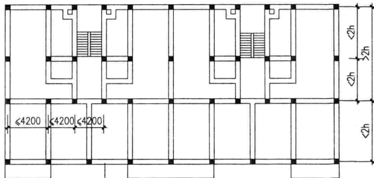
构造柱布置示意图 3
