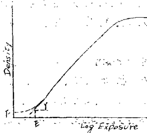
图 1.1 赫德特性曲线
