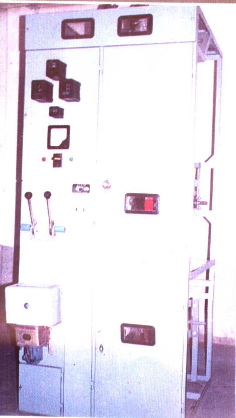
重庆金华电器成套公司生产的GG-1A(下)高压柜
