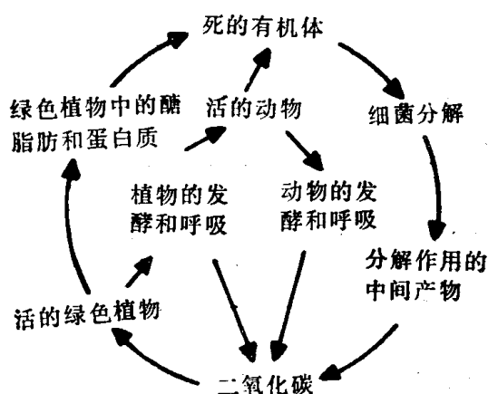
图2-1 自然界中碳的循环
