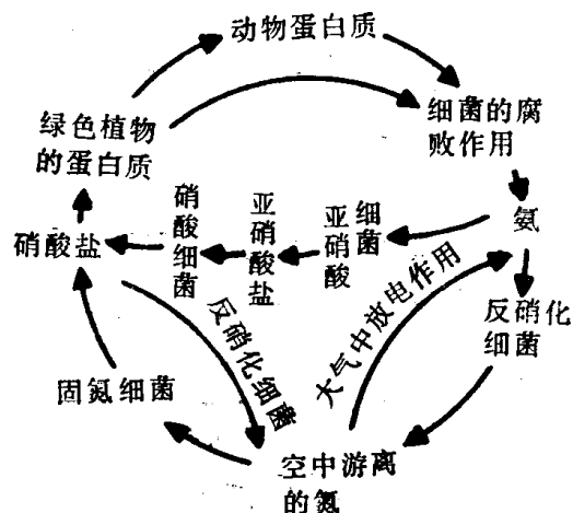
图2-2 自然界中氮的循环
