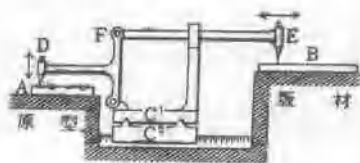
圖 1.1.4 浮彫影刻機之原理。
